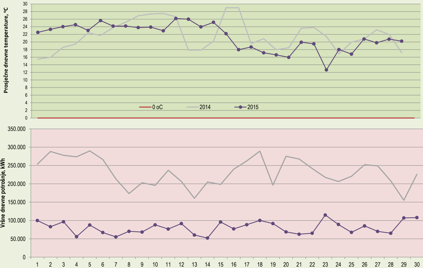
Dijagram potrošnje kućanstava (kWh) u ovisnosti o T_{sr} °C na MRS Vinkovci LIPANJ 2014 i 2015
