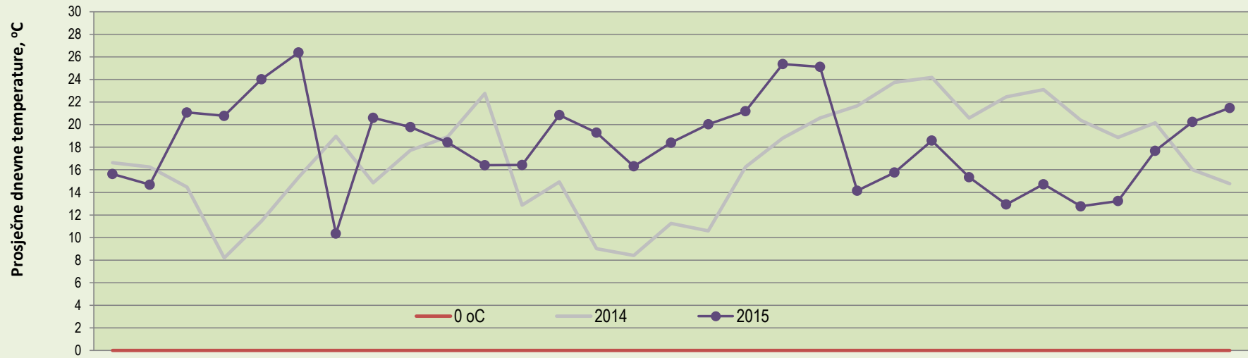
Dijagram potrošnje kućanstava (kWh) u ovisnosti o T_{sr} °C na MRS Vinkovci SVIBANJ 2014 i 2015
