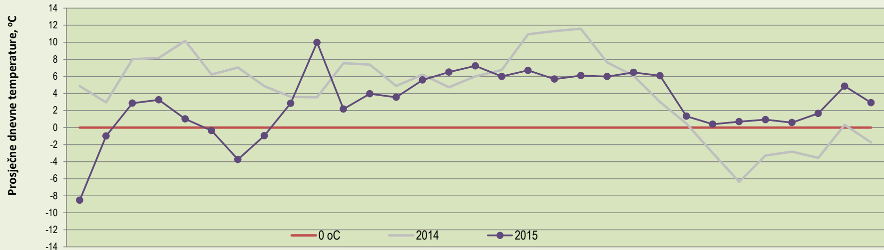
Dijagram potrošnje kućanstava (kWh) u ovisnosti o T_{sr} °C na MRS Vinkovci SIJEČANJ 2014 i 2015
