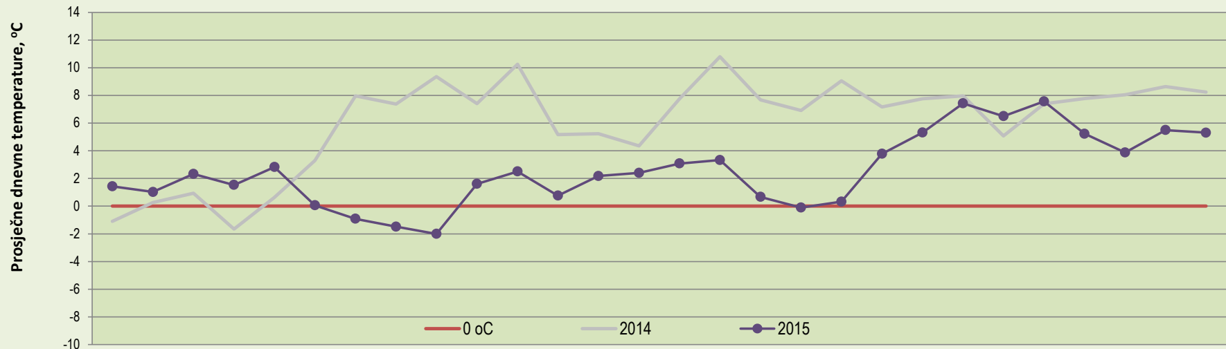
Dijagram potrošnje kućanstava (kWh) u ovisnosti o T_{sr} °C na MRS Vinkovci VELJAČA 2014 i 2015
