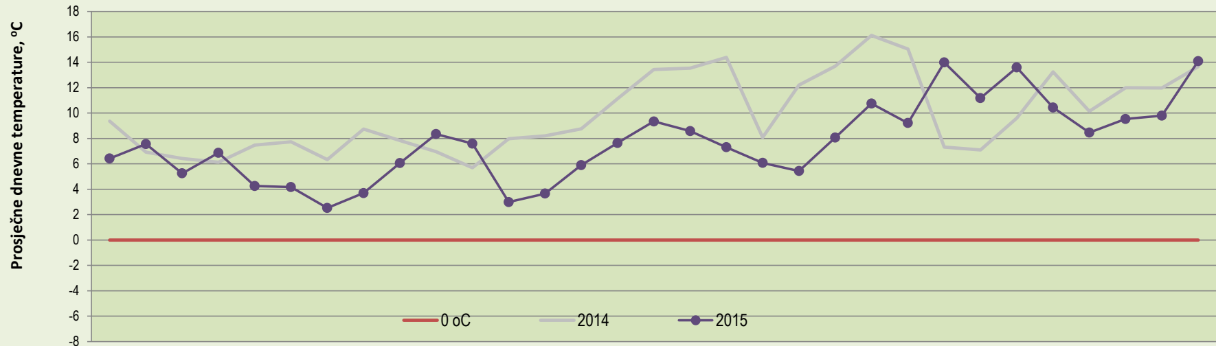
Dijagram potrošnje kućanstava (kWh) u ovisnosti o T_{sr} °C na MRS Vinkovci OŽUJAK 2014 i 2015
