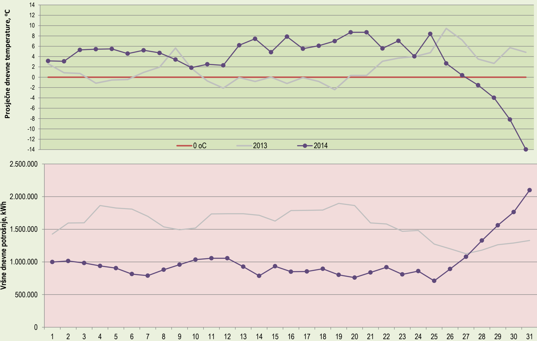
Dijagram potrošnje kućanstava (kWh) u ovisnosti o T_{sr} °C na MRS Vinkovci PROSINAC 2013 i 2014
