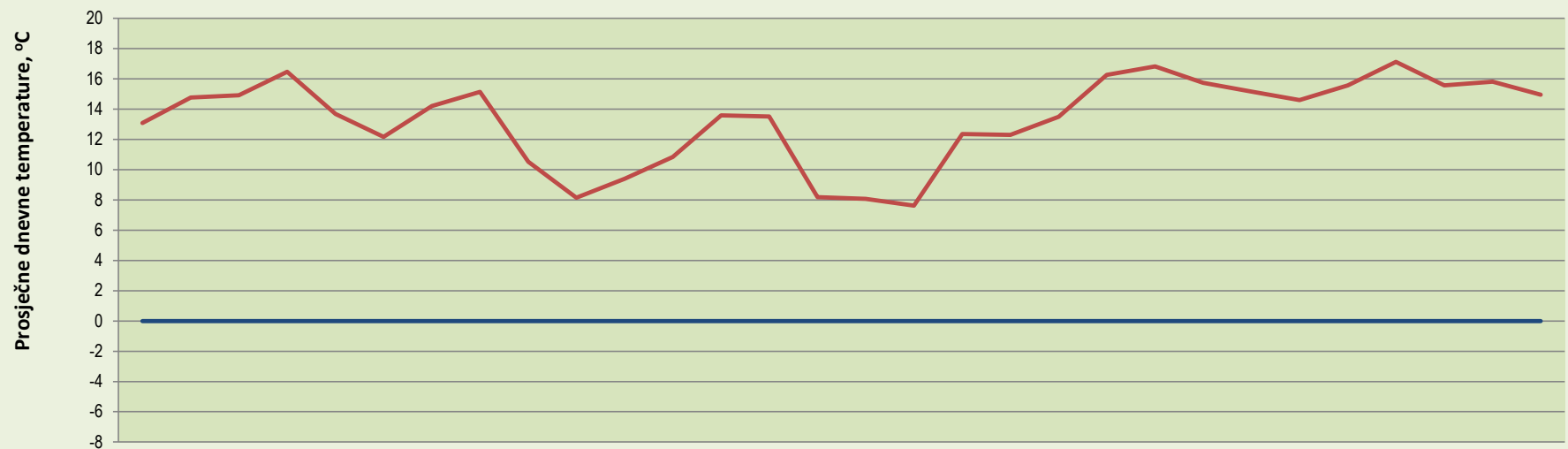
Dijagram ovisnosti ukupne potrošnje o prosječnim dnevnim temperaturama na MRS Vinkovci - mjerenje ODS TRAVANJ 2014
