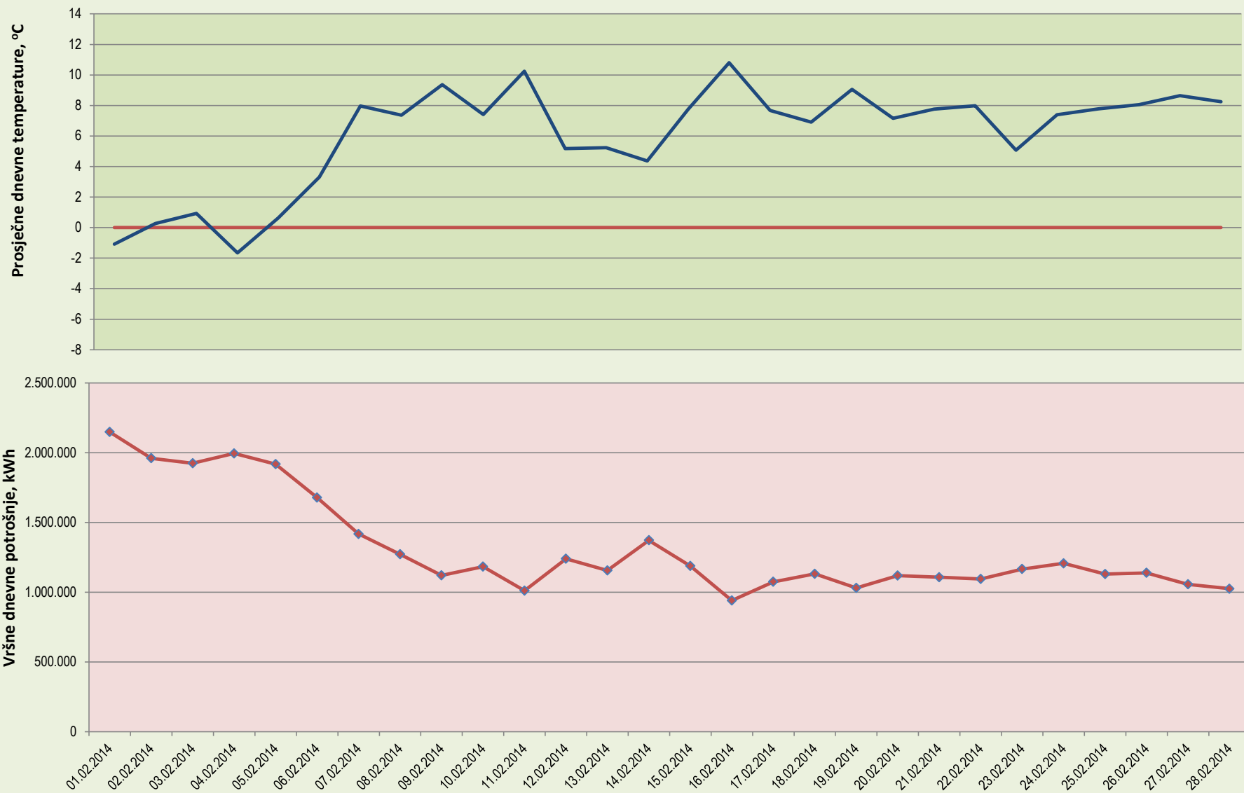
Dijagram ovisnosti ukupne potrošnje o prosječnim dnevnim temperaturama na MRS Vinkovci - mjerenje ODS VELJAČA 2014
