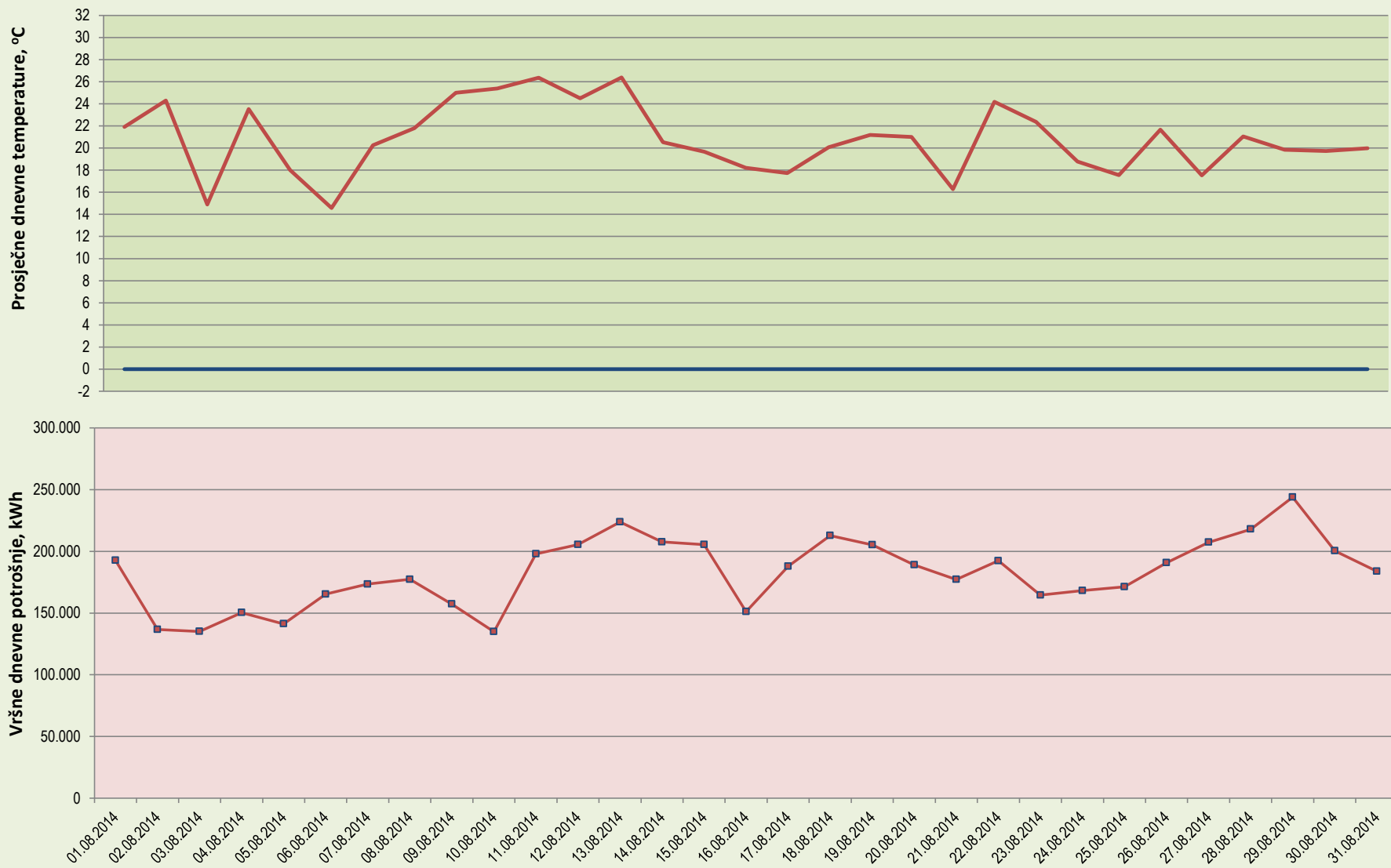
Dijagram ovisnosti ukupne potrošnje o prosječnim dnevnim temperaturama na MRS Vinkovci - mjerenje ODS KOLOVOZ 2014
